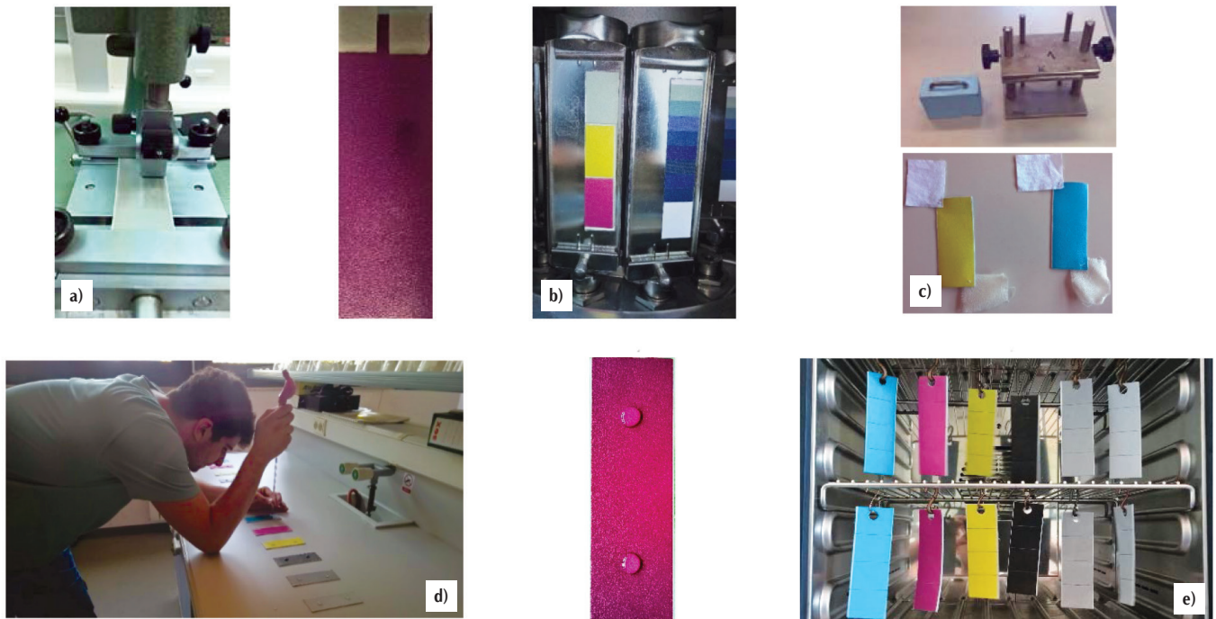
Slika 2. Ispitivanje postojanosti otiska na: a) suho i mokro trljanje, b) djelovanje umjetnog svjetla, c) djelovanje vode, d) vodene kapi, e) ubrzano starenje djelovanjem topline
